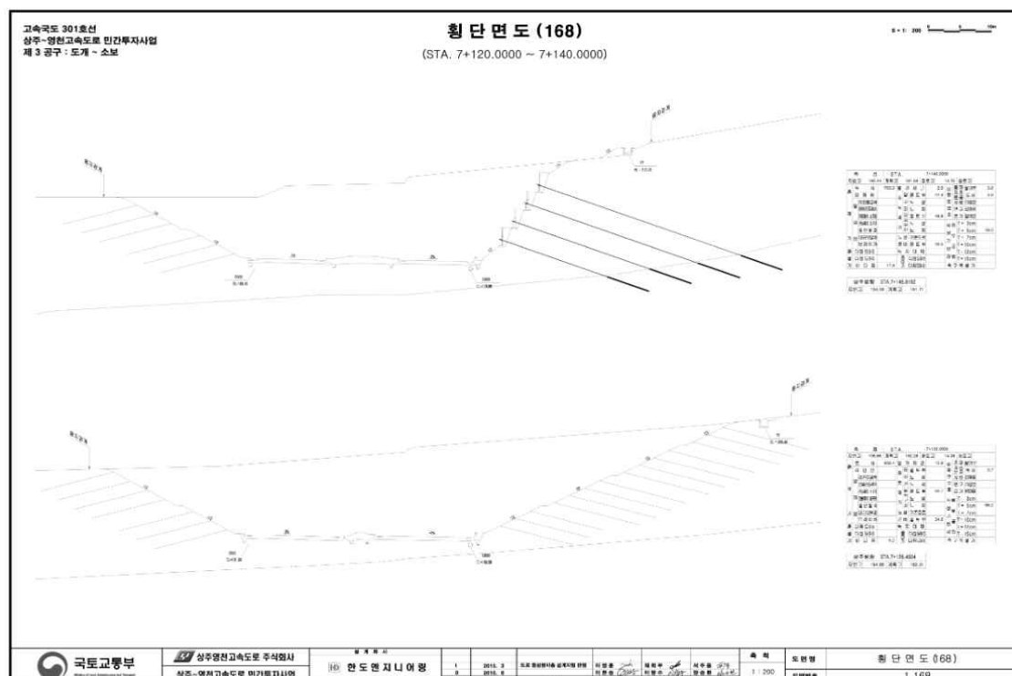
【그림 18.1.5】 표준횡단면도
